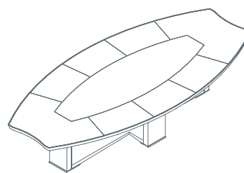
Tavolo meeting forma ellittica 1IA4611: L 280 P 145 H 72 1IA4612: L 350 P 165 H 72 1IA4613: L 420 P 180 H 72
